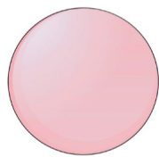
Kugle
