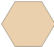
Sekskant
