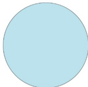
Cirkel
