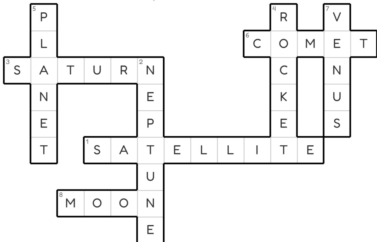
Neptun
