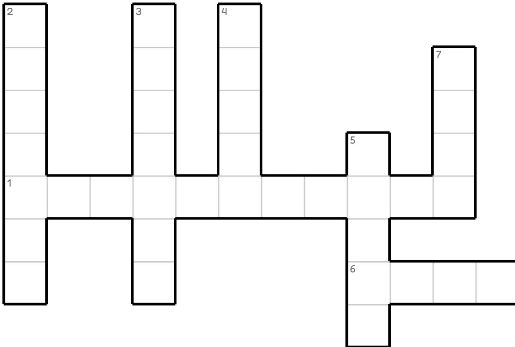
Haystack
