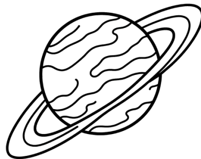
planet
