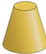
Cone
