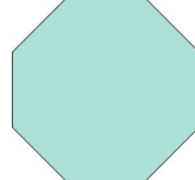
Octogon
