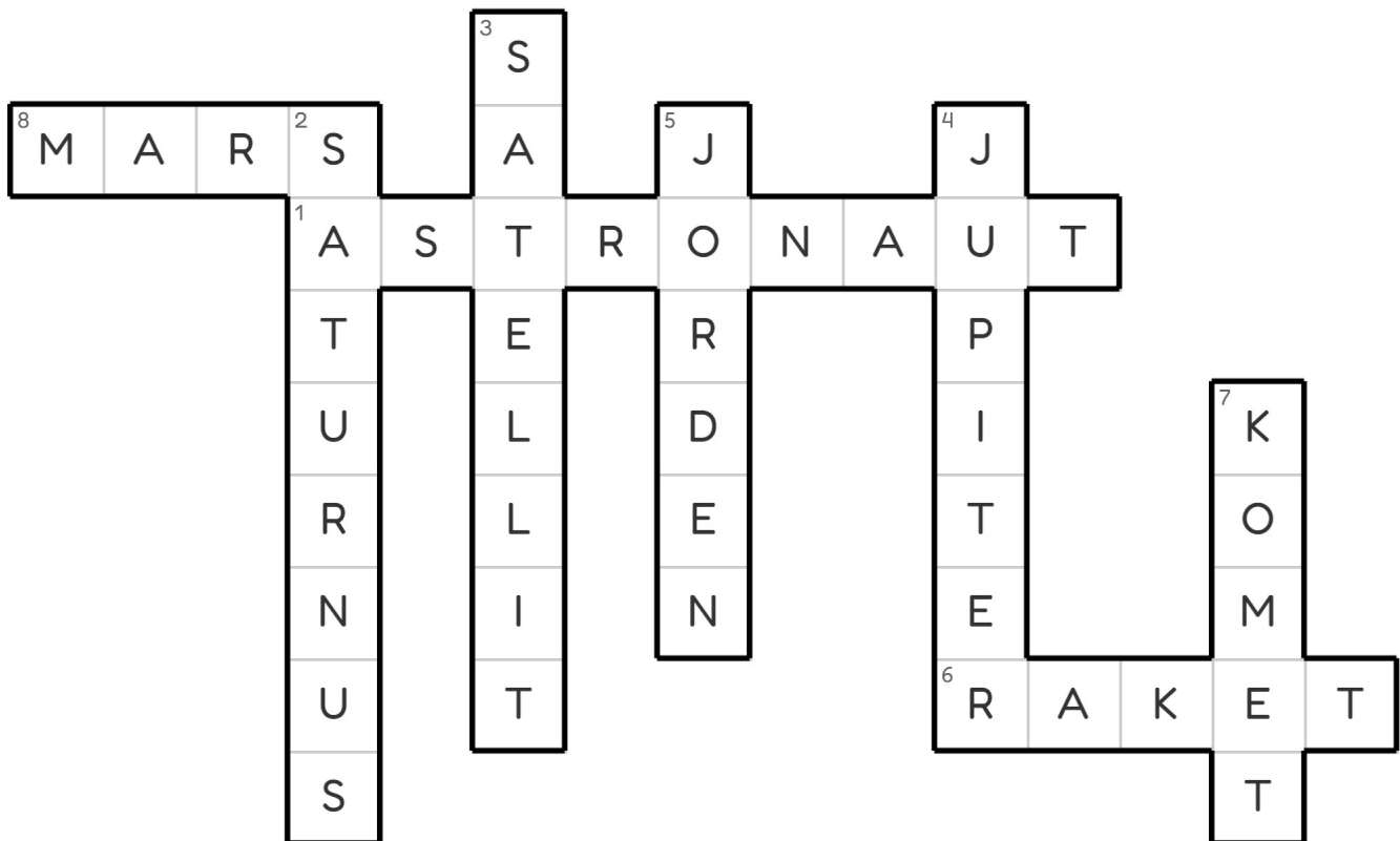
Jupiter
