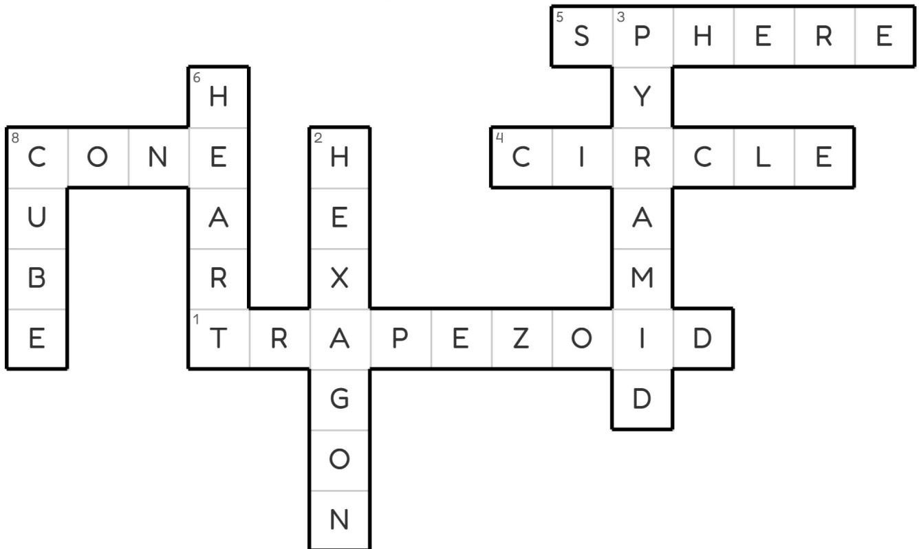
Trapezio
