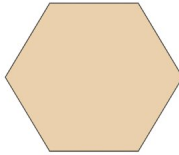
Hexágono
