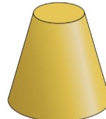
Cono
