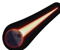
meteoro
