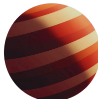
venus
