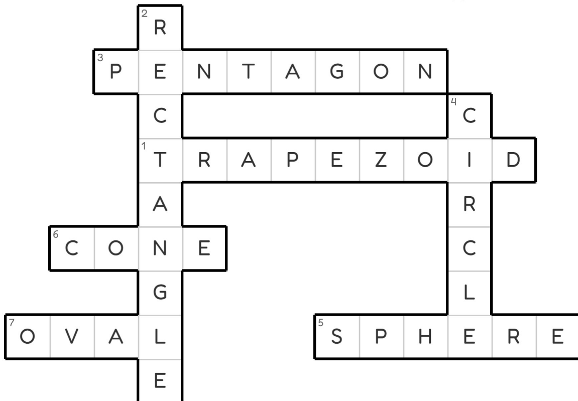
Ympyrä
