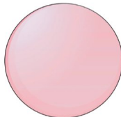
Pallo
