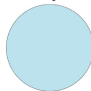
Ympyrä
