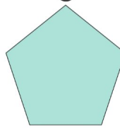
Viisikulmio
