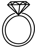
vinoneliö
