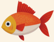
poisson
