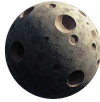
astéroïde
