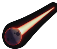
météore
