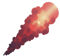
comète
