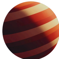
vénus
