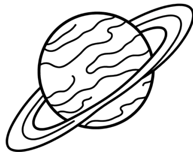
pianeta
