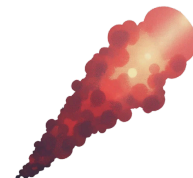
cometa
