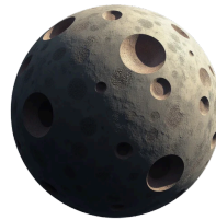
asteroïde
