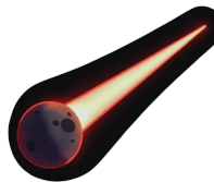
meteoor
