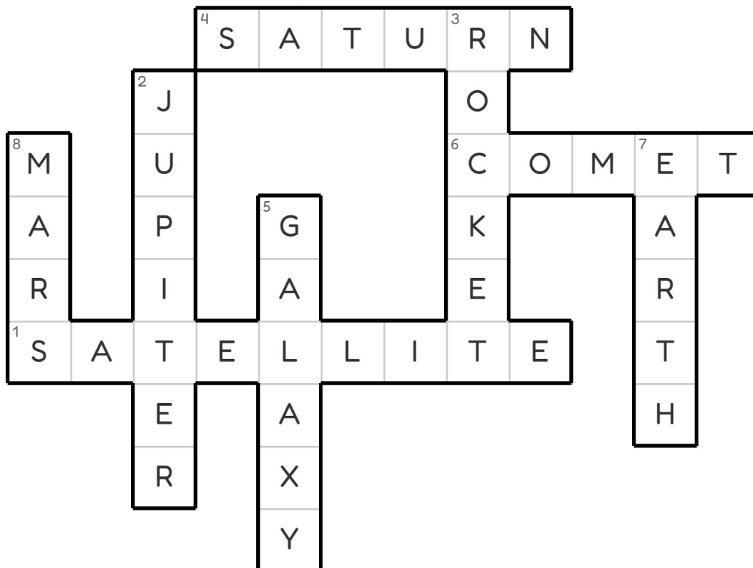
Jupiter
