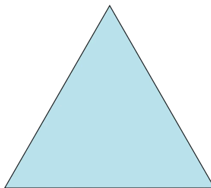
triângulo
