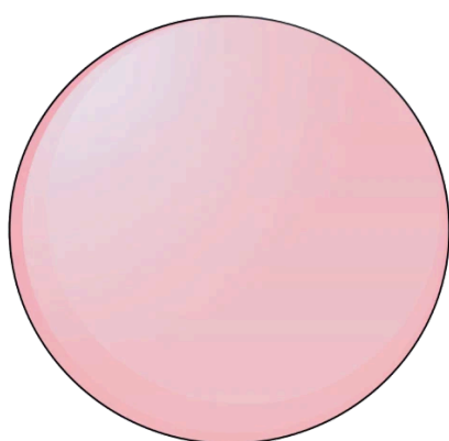
esfera
