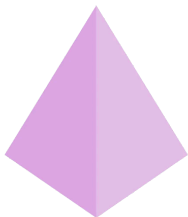
pirâmide
