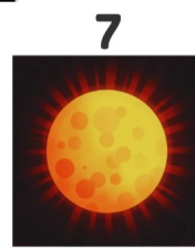
Sol
