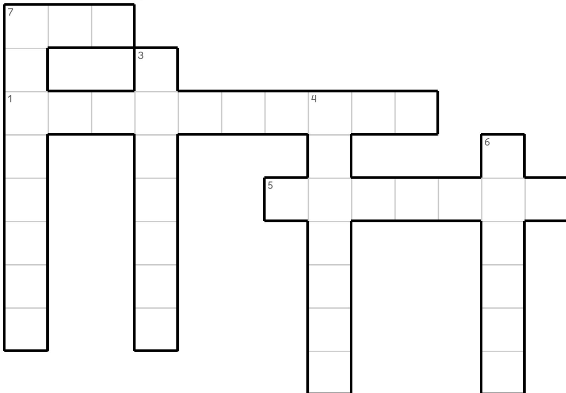
Telescópio
