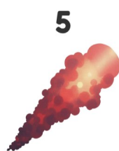
Cometa
