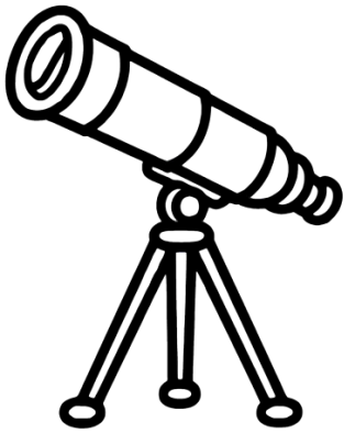
teleskop
