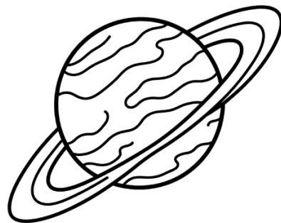
planet
