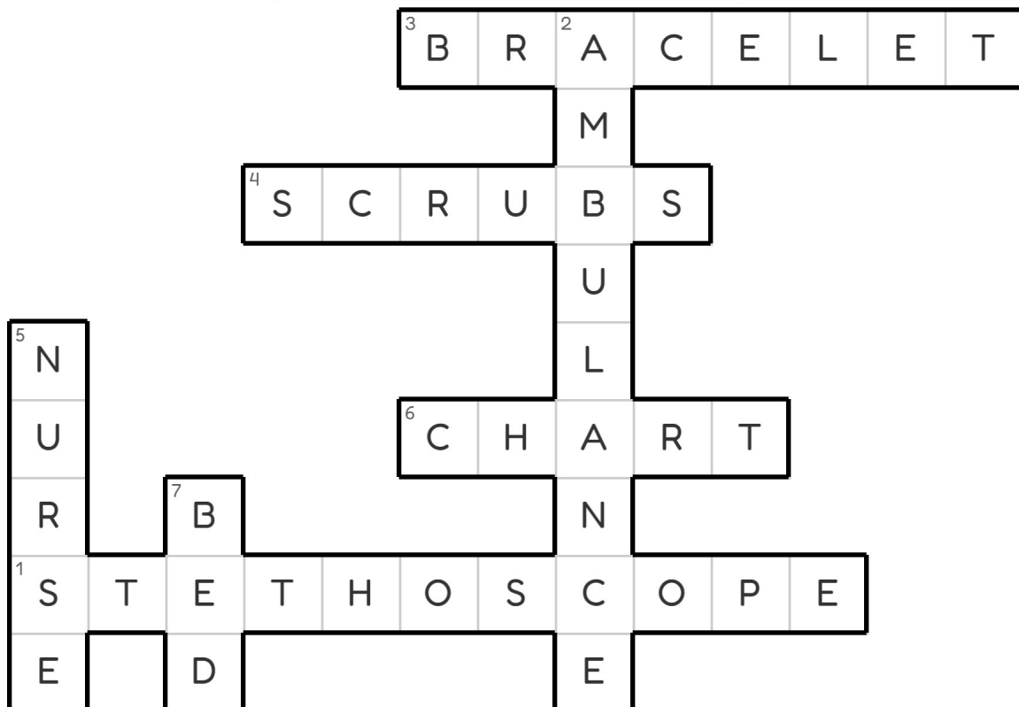
1 Stetoskop
